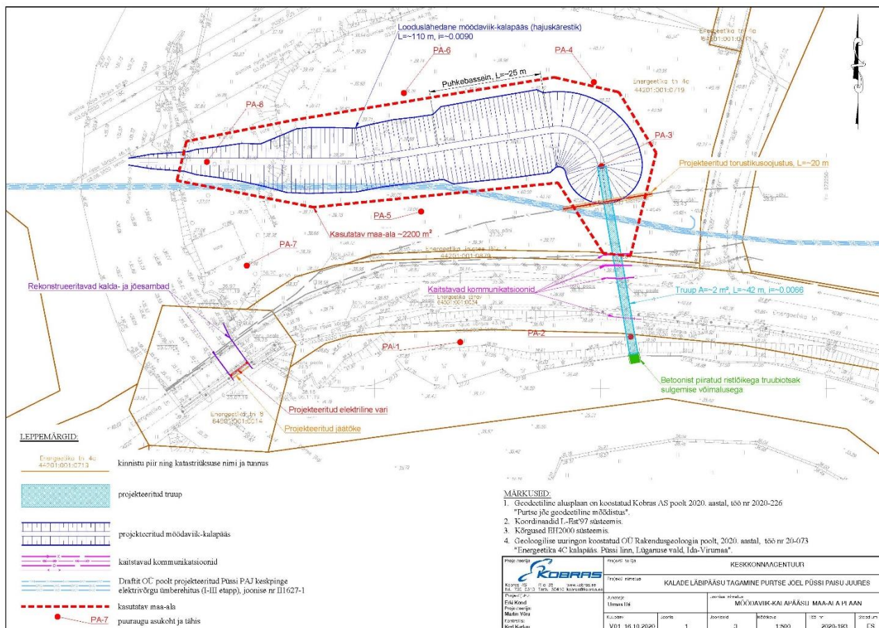
Joonis 3. Möödaviik-kalapääsu variant (Kobras AS, 2020).
