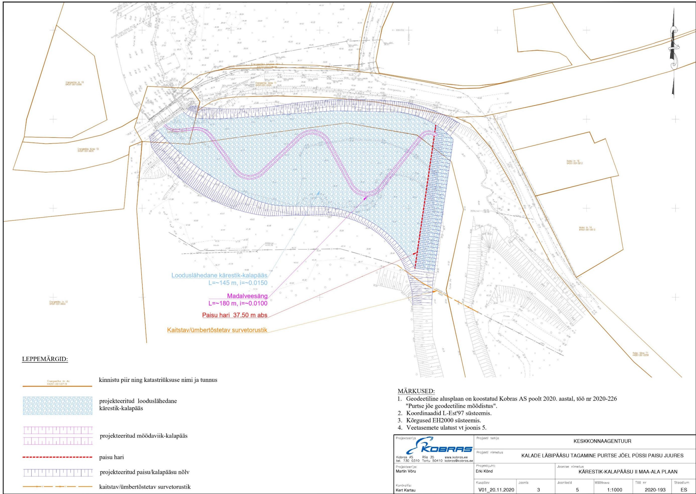
Joonis 6. Käreistik-kalapääsu II maa-ala plaan (Kalade läbipääsu tagamine Purtse jõel Püssi paisu juures, töö nr 2020-193, 2020).
