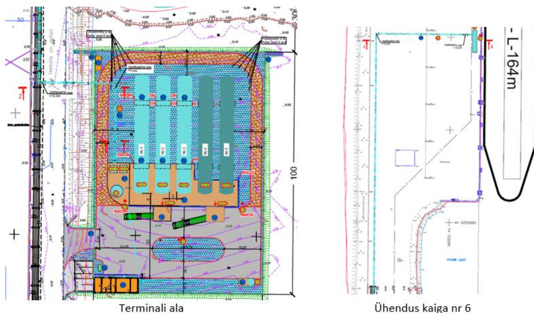
Joonis 2.1. Kavandatava terminali seadmete paiknemine
